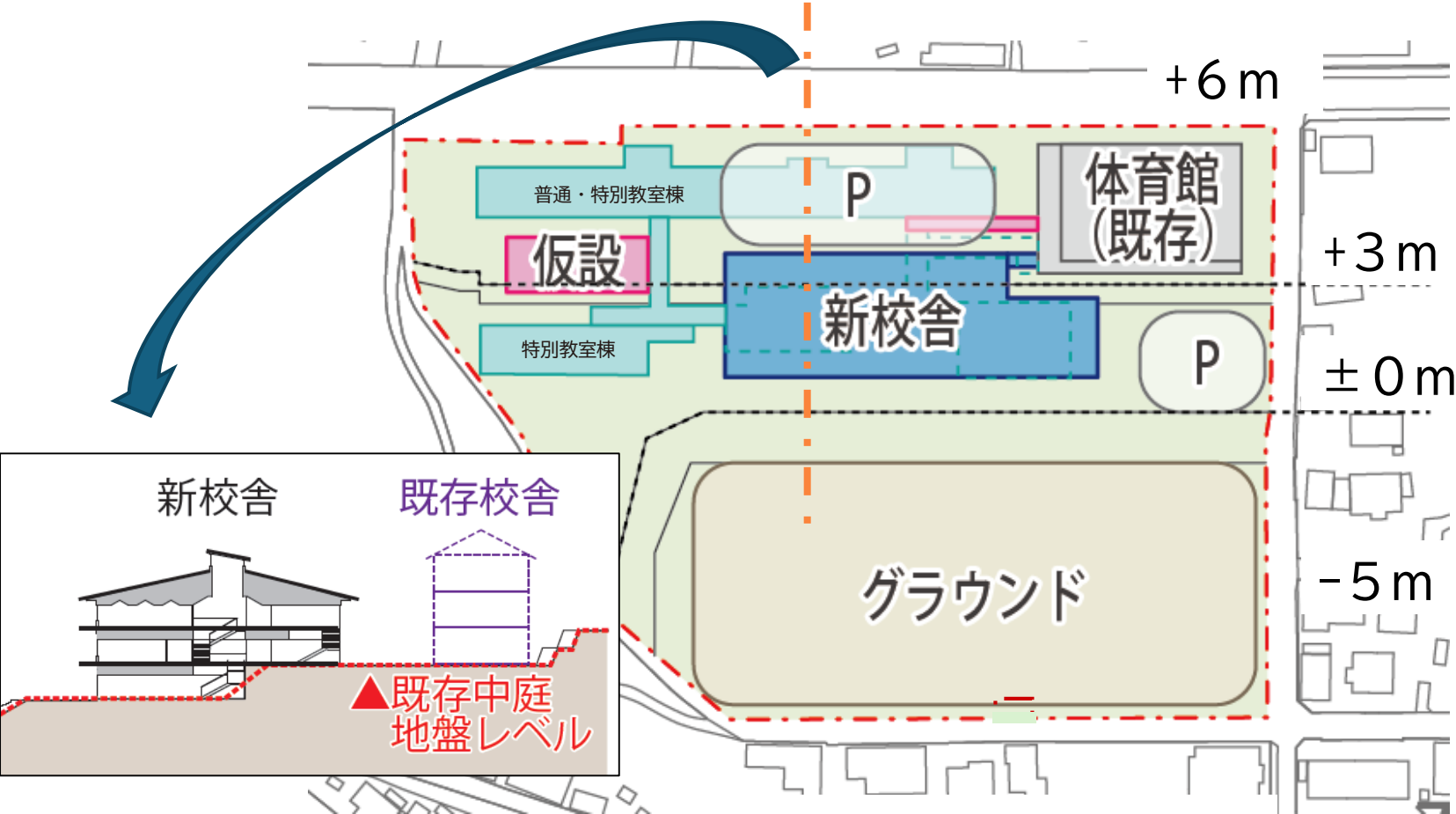
建物配置計画（案）
