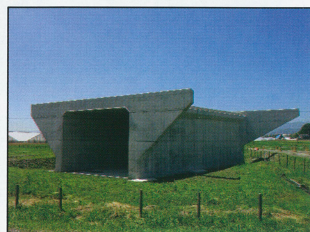
8号函渠
