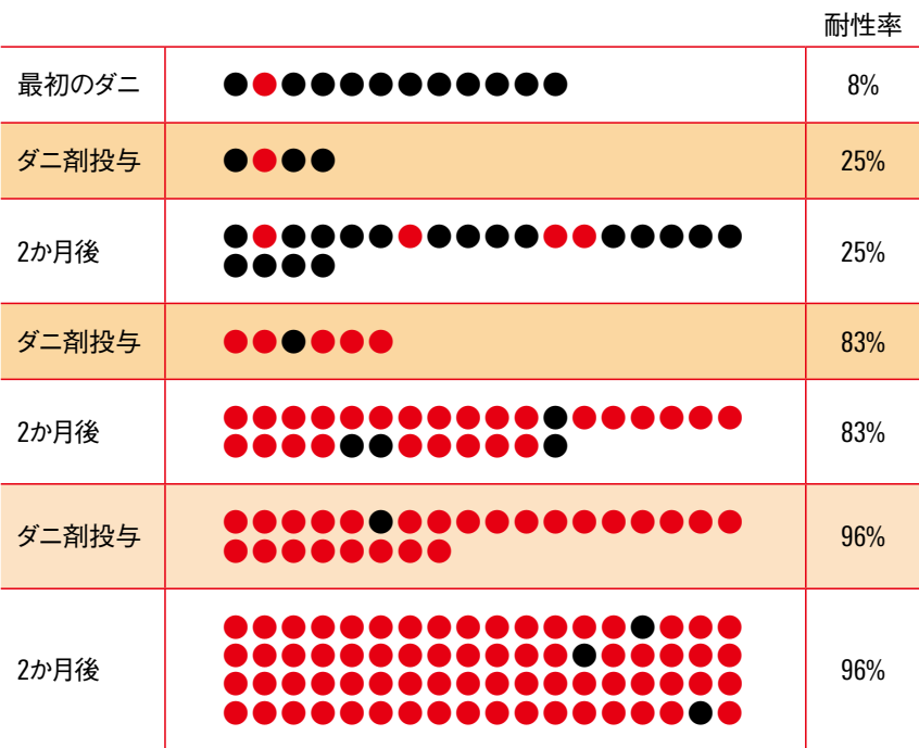
図20 抵抗性のダニが増加するメカニズム 赤色の丸は抵抗性のダニを示す
