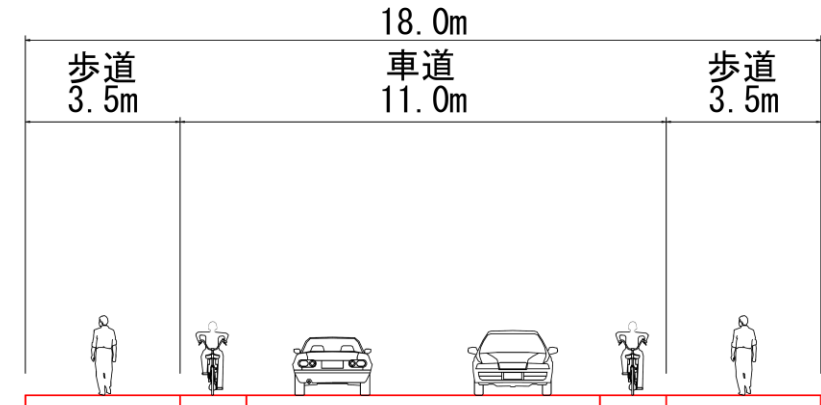
標準断面図
