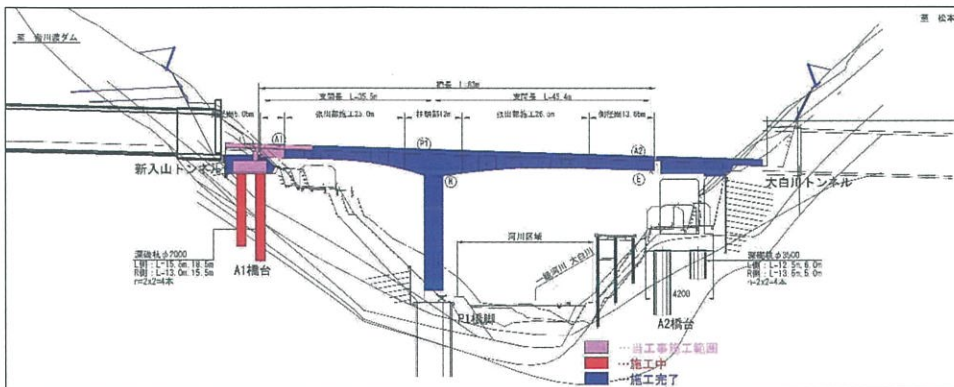
大白川大橋 側面図
