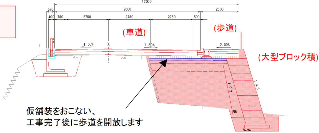
B - B' 断面
