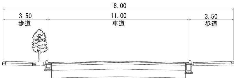
標準断面図
