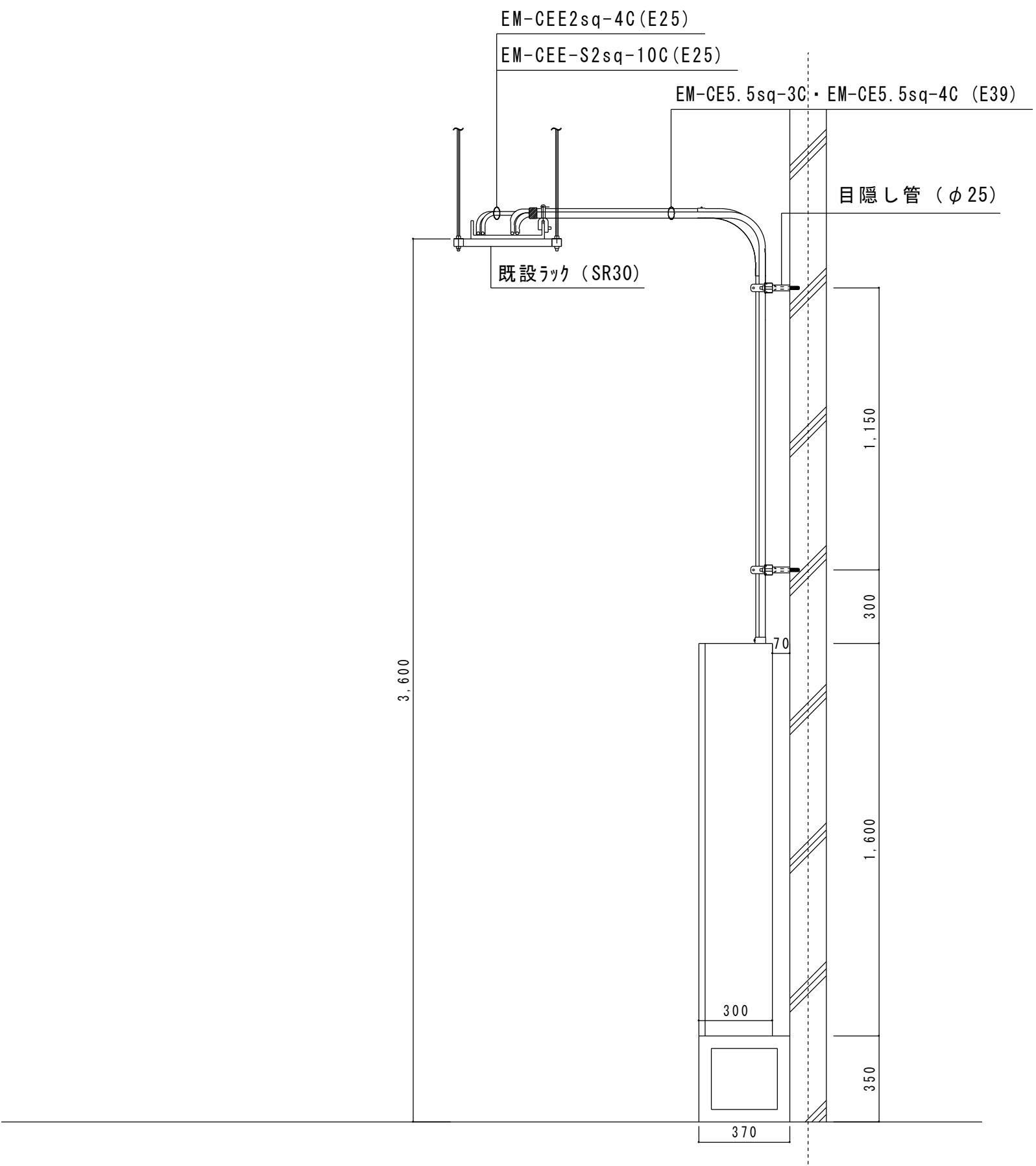
機械室 井戸ポンプ制御盤配管・配線標準図 (1/20)
