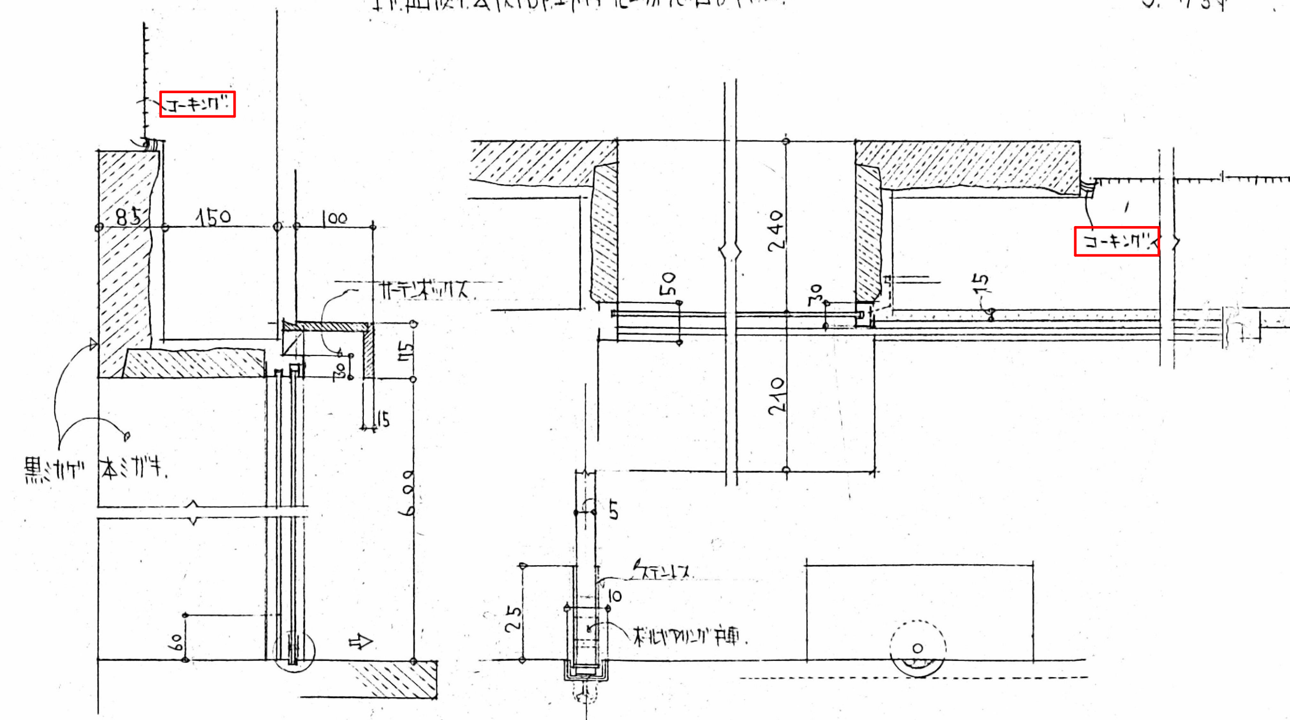
1. 西側玄關門外付売場窓口詳細.
