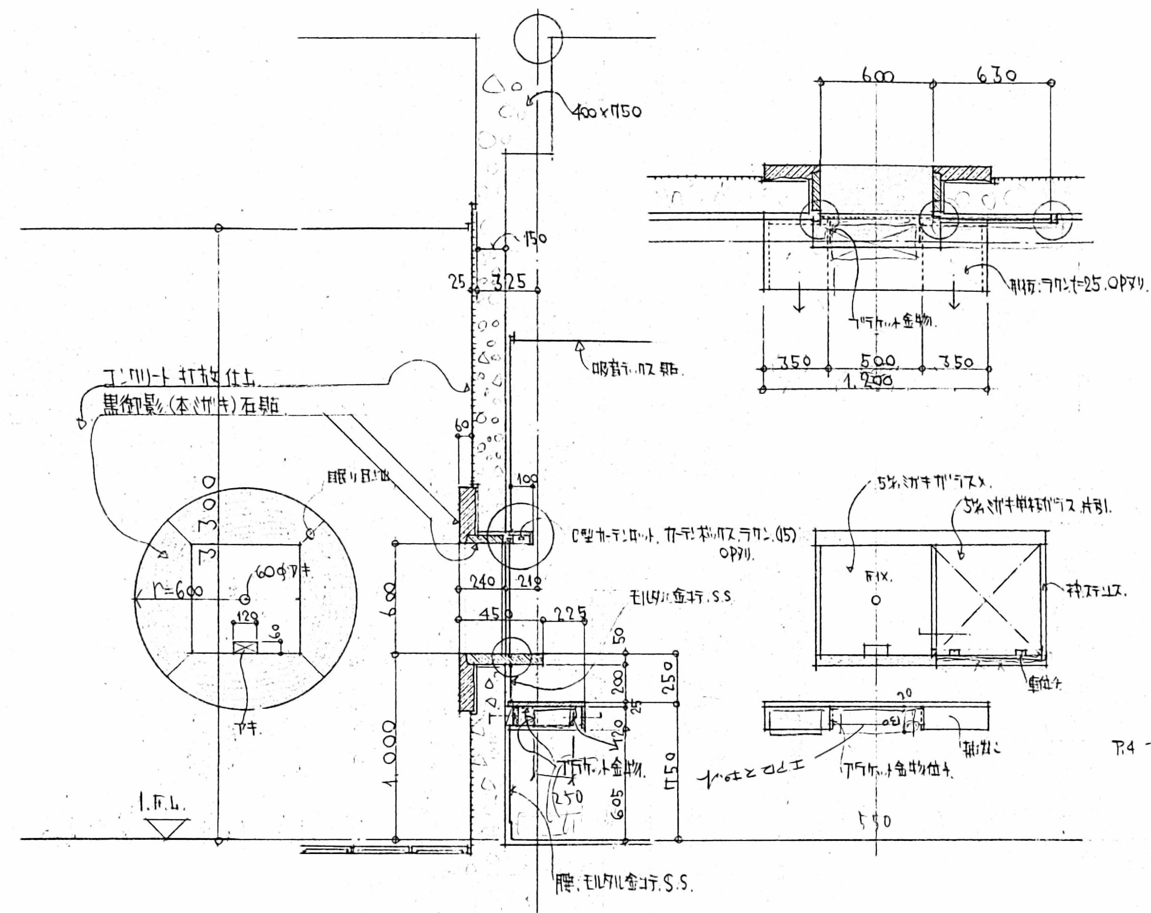
1. 西側玄關門外付売場窓口詳細.
