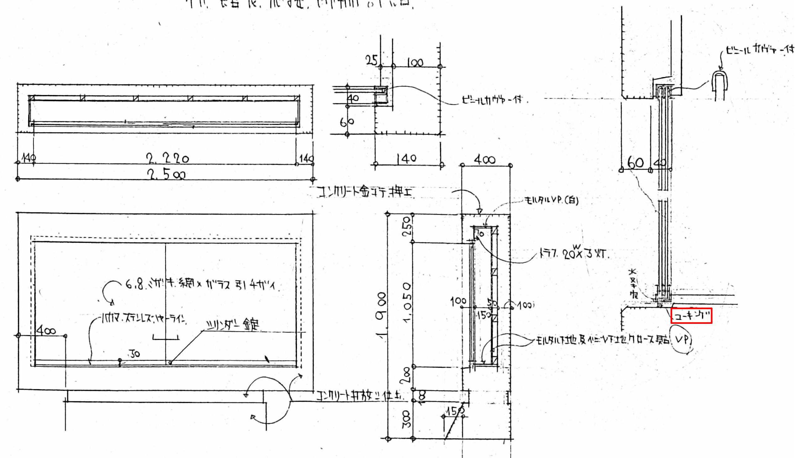
揭示板註釋 S. 1/20
