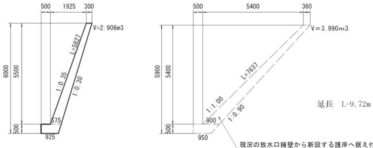
コンクリート擁壁工断面図
