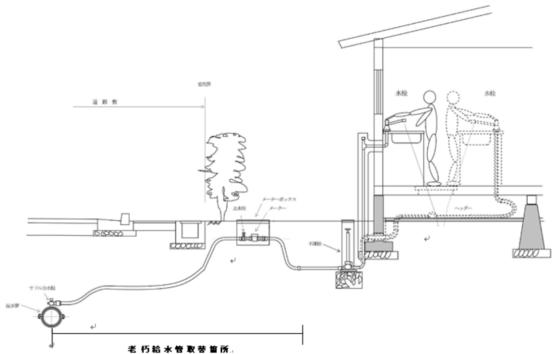
老朽給水管取替業務の施工範囲
