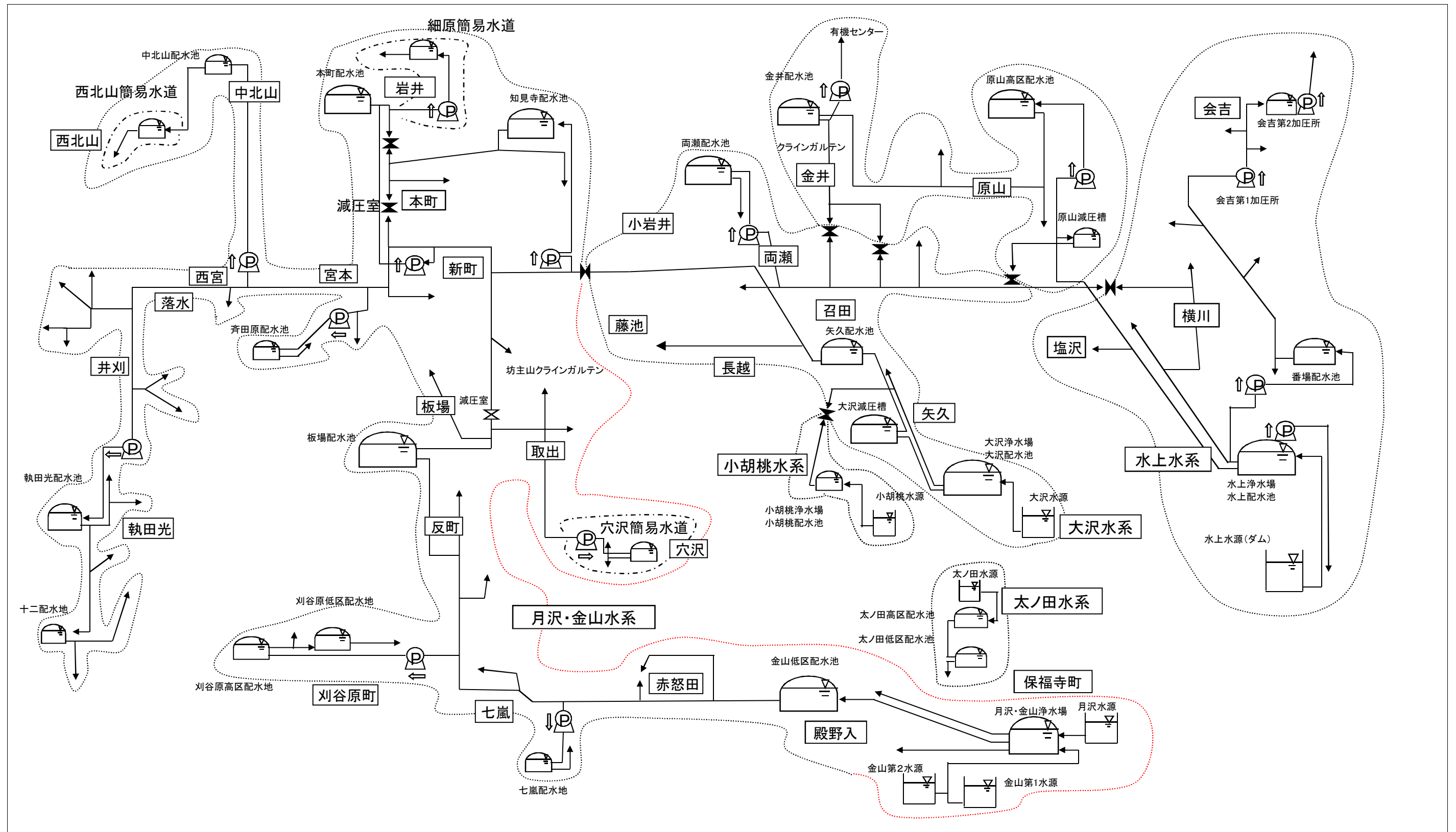
(2) 四賀地区配水系統概要図
