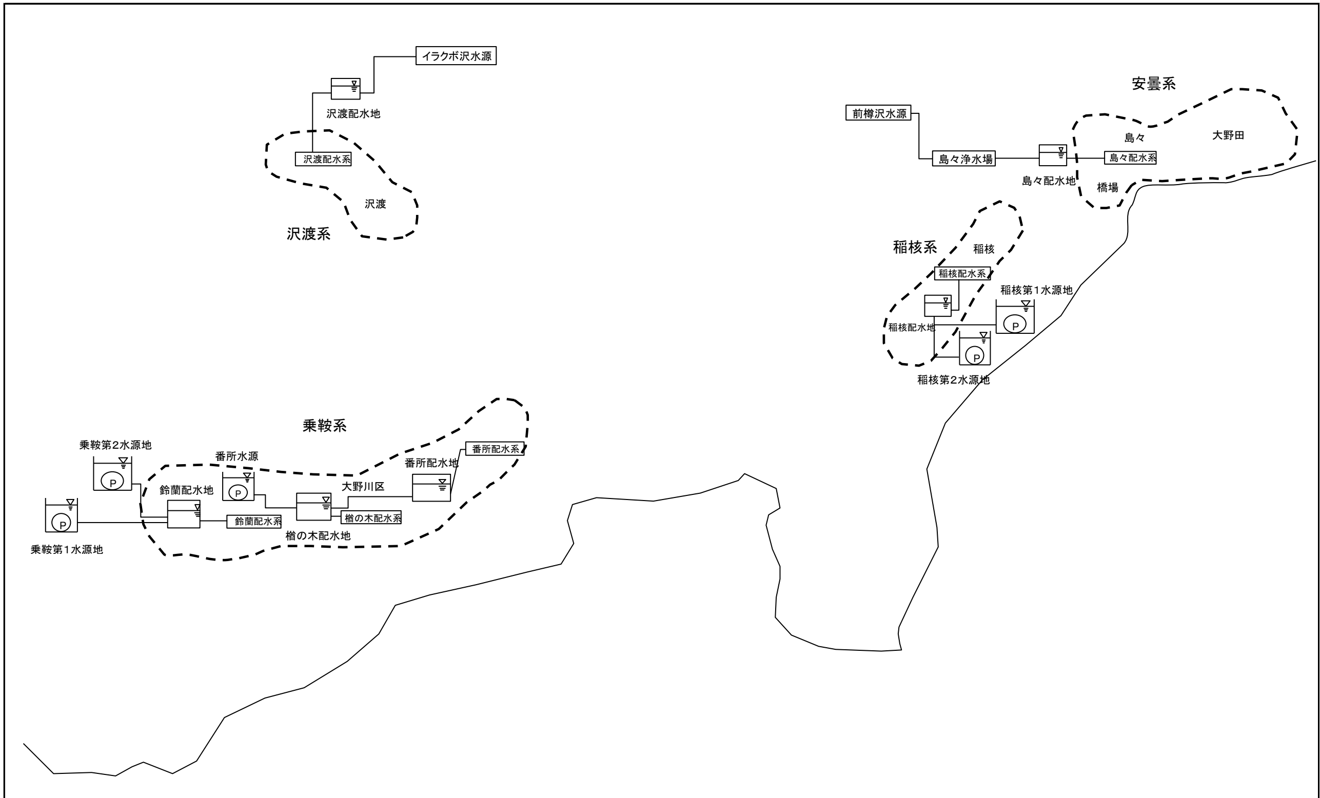
(3-2) 梓川地区水道事業(安曇)配水系統概要図
