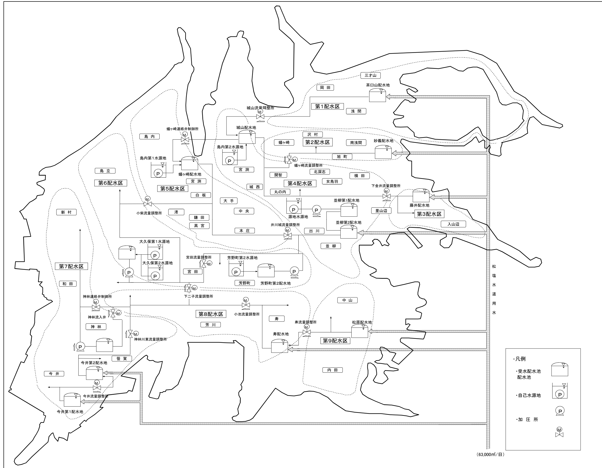
(1) 松本地区配水系統概要図
