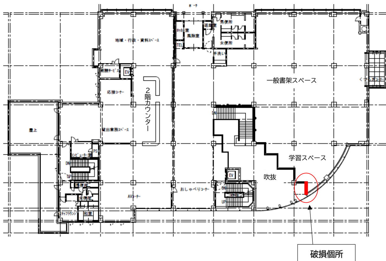
配置図 (2階)
