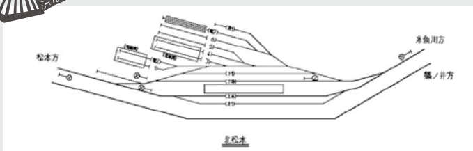
線路配線図 昭和53年(1978年)12月25日
