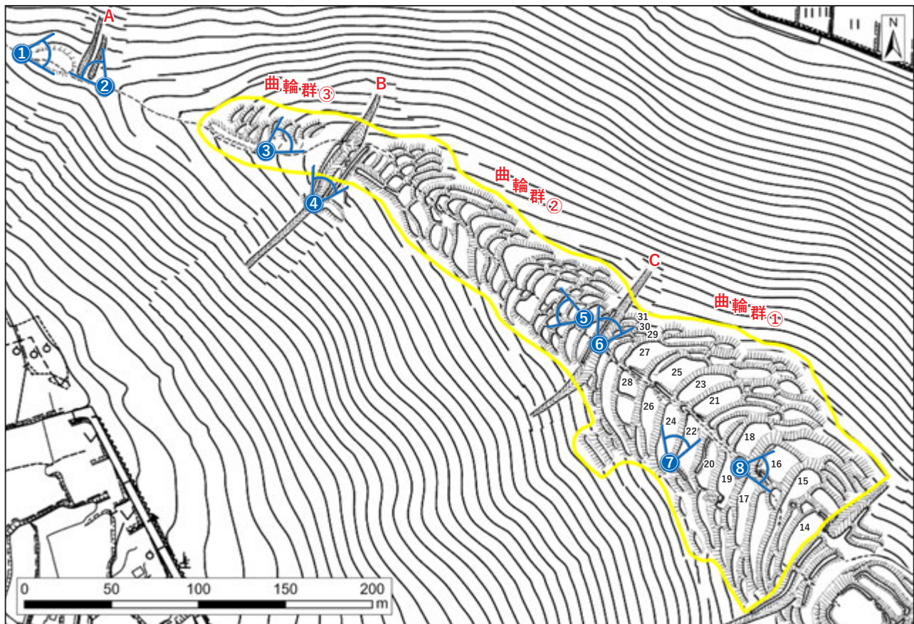
【図 32】 大城 西北西尾根ブロック拡大図
