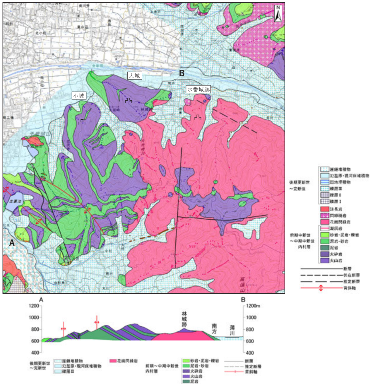
【図19】林城跡周辺地質図と断面図（小山俊滉氏作製図を一部加工）
