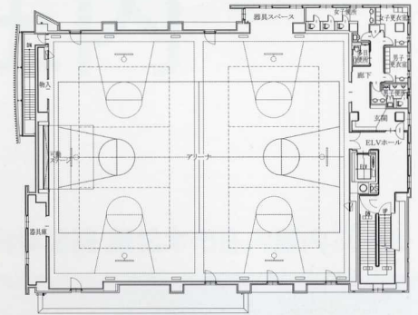
4階平面図
