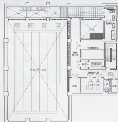
地下1階平面図
