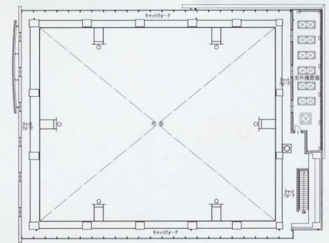
4階平面図
