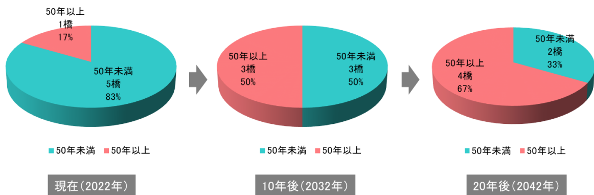
図 1.1 横断歩道橋の経過年推移
