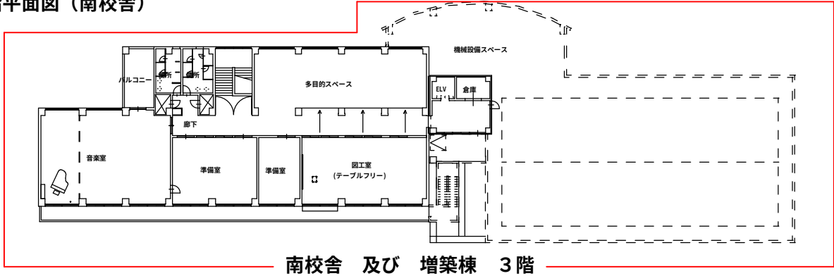
3 階平面図 (南校舎)
