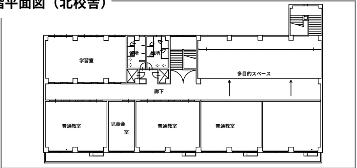
2階平面図
