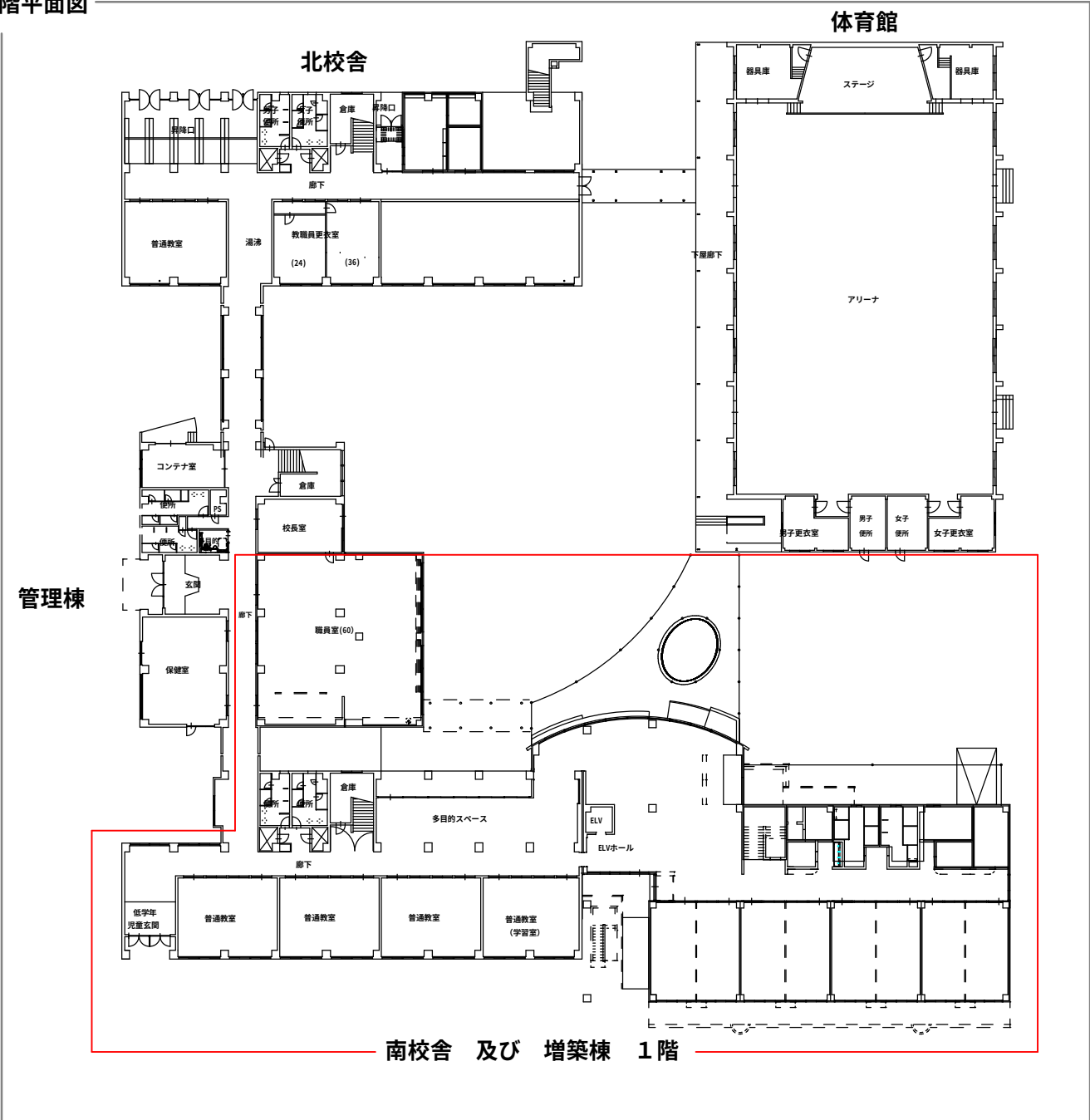
1階平面図
