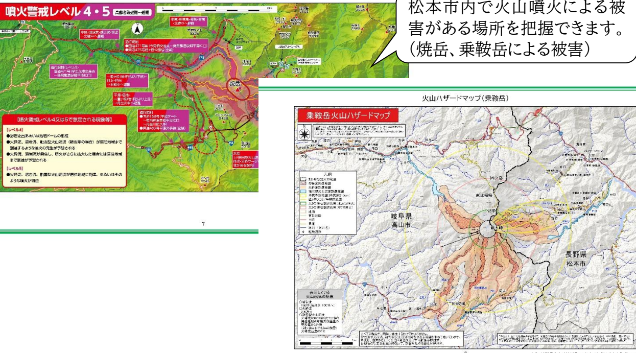
火山ハザードマップ(焼岳)
