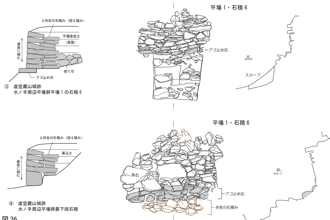
図 26 虚空蔵山城跡の石積断面模式図
