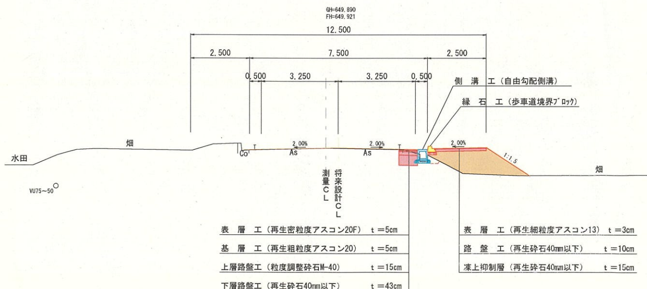
標準横断図
