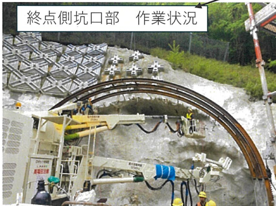
■ 終点側坑口部 支保工設置作業状況
