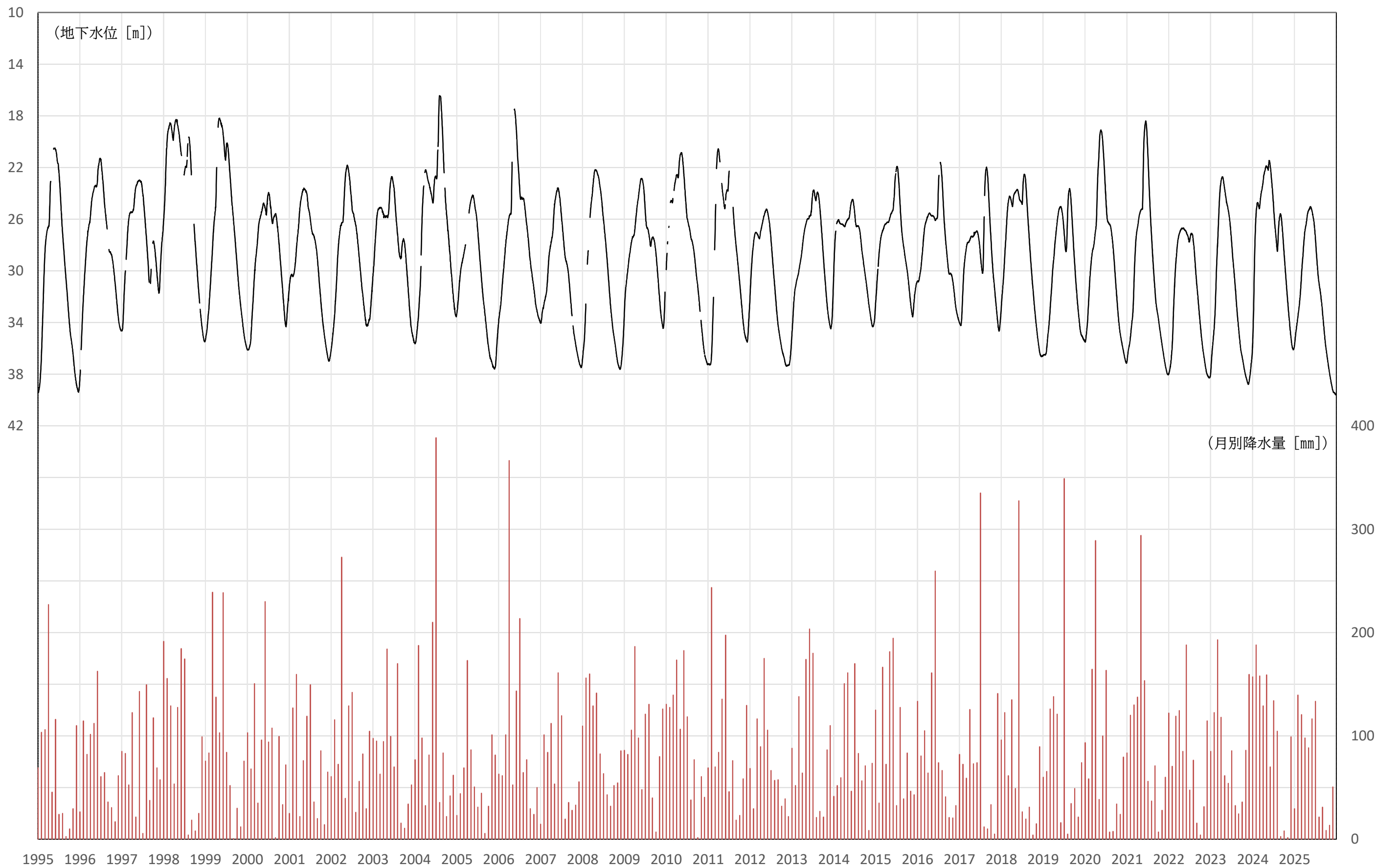
経年地下水位観測図 <今井観測井>
