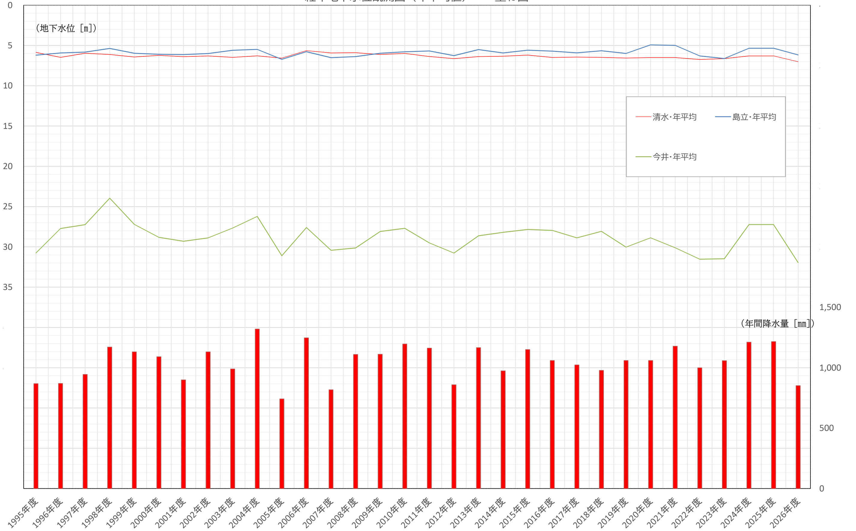
経年地下水位観測図（年平均値） <重ね図>
