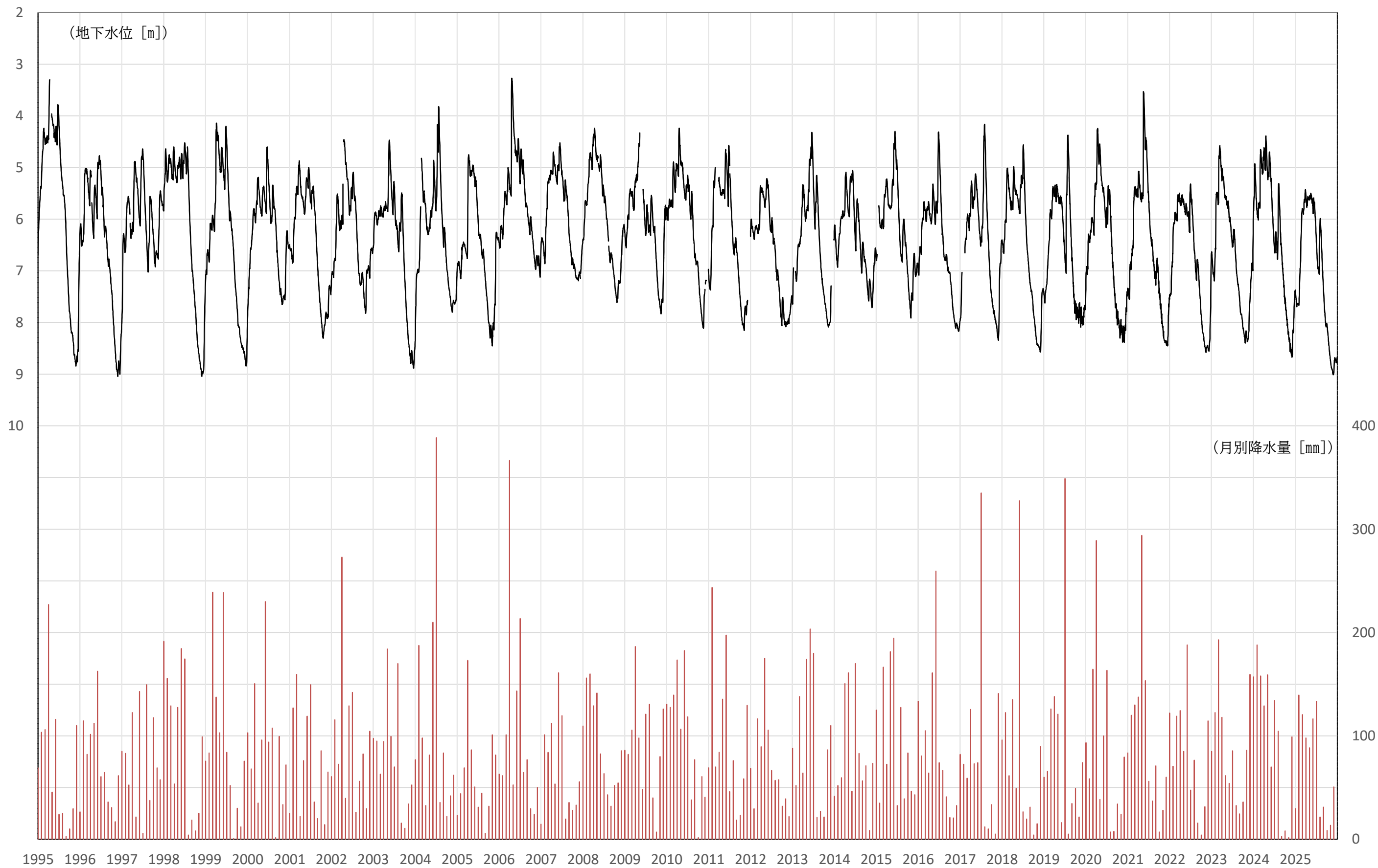
経年地下水位観測図 <清水観測井>
