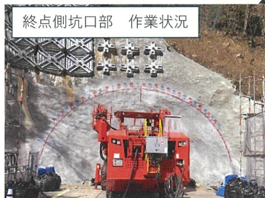
■終点側坑口部 トンネル補助工法を施工中
