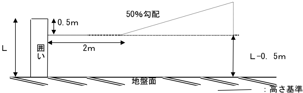
図2 囲いに接して廃棄物を保管しようとする場合
