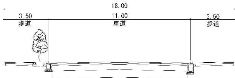
標準断面図
