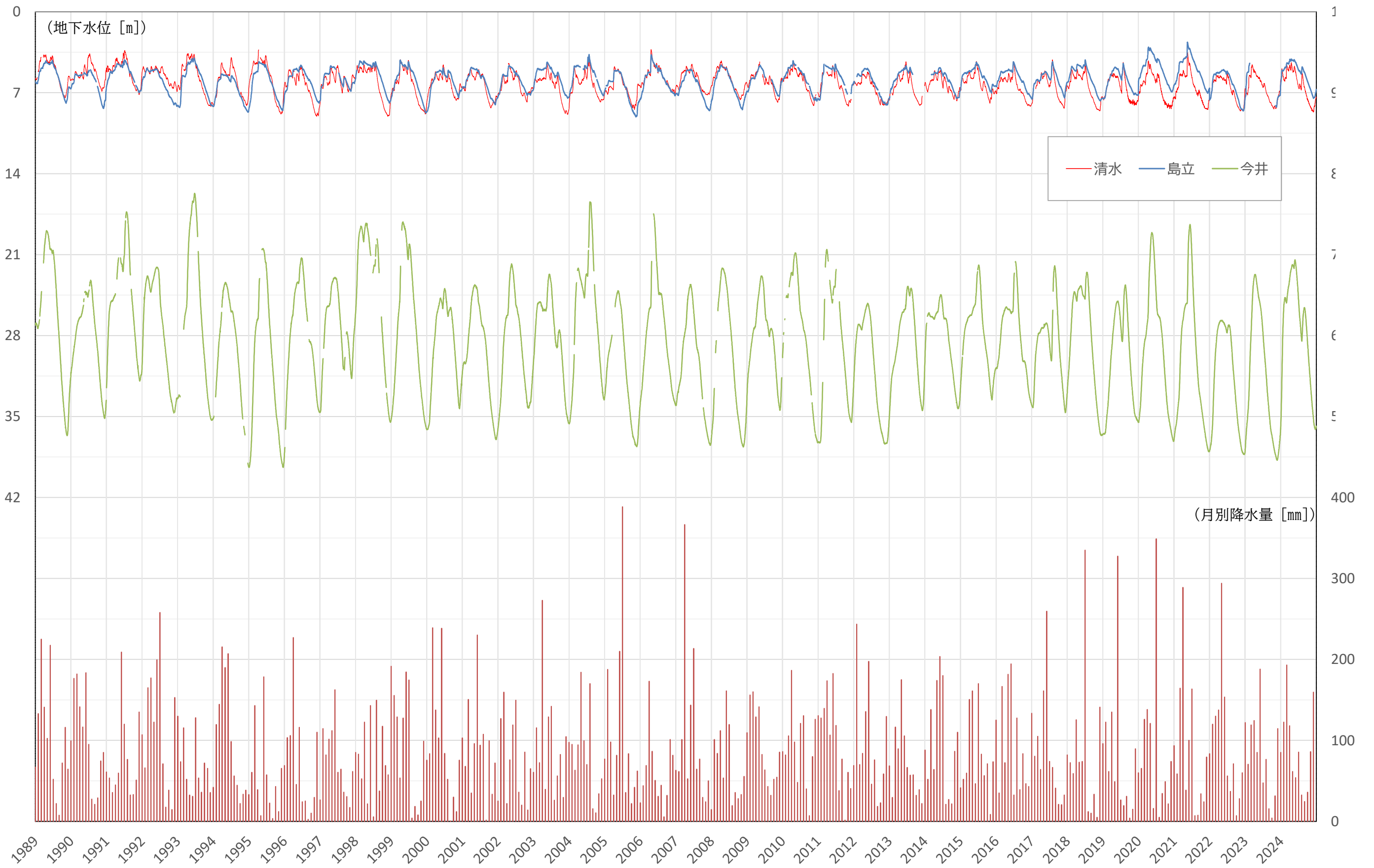
経年地下水位観測図 <重ね図>
