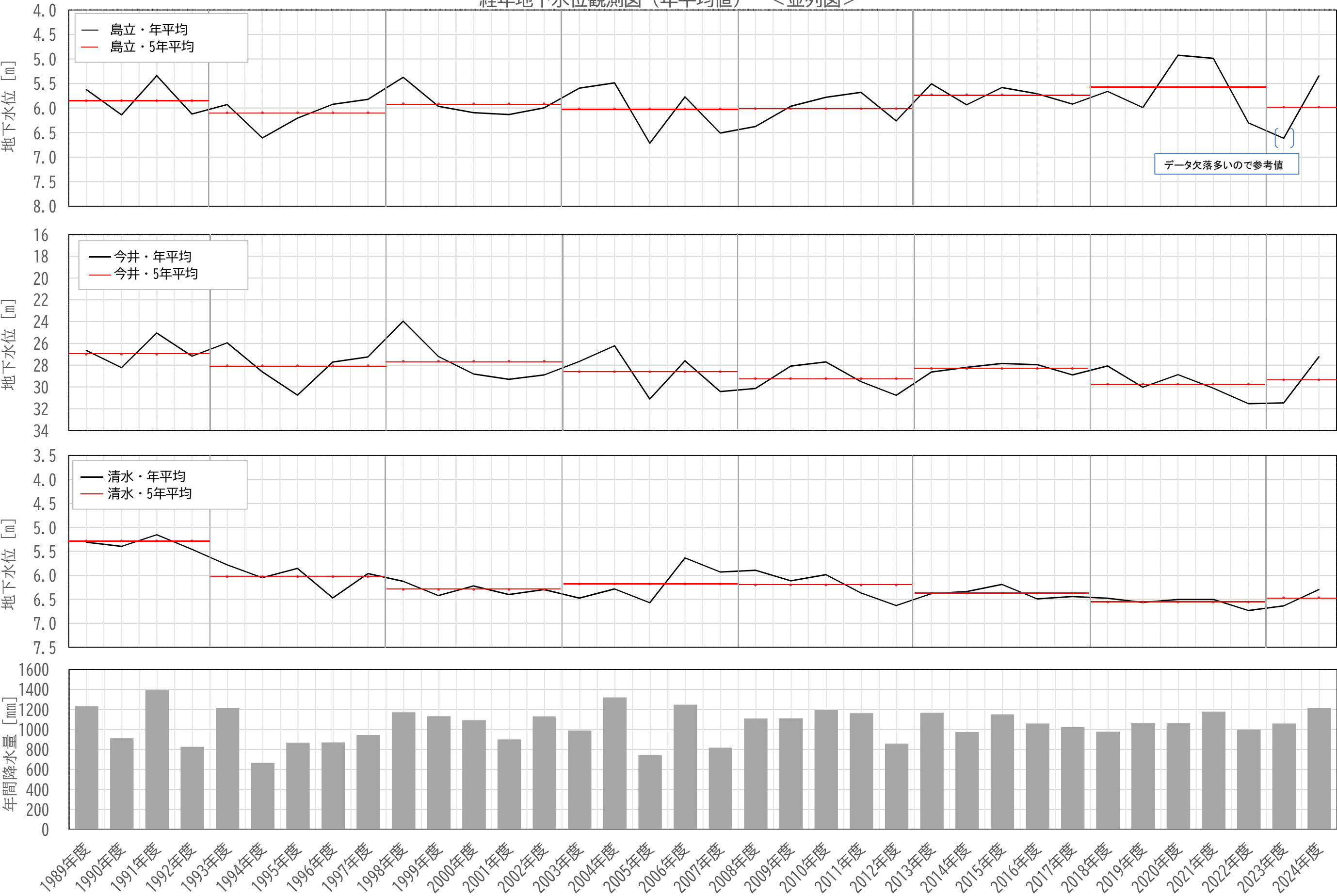
経年地下水位観測図（年平均値） <並列図>
