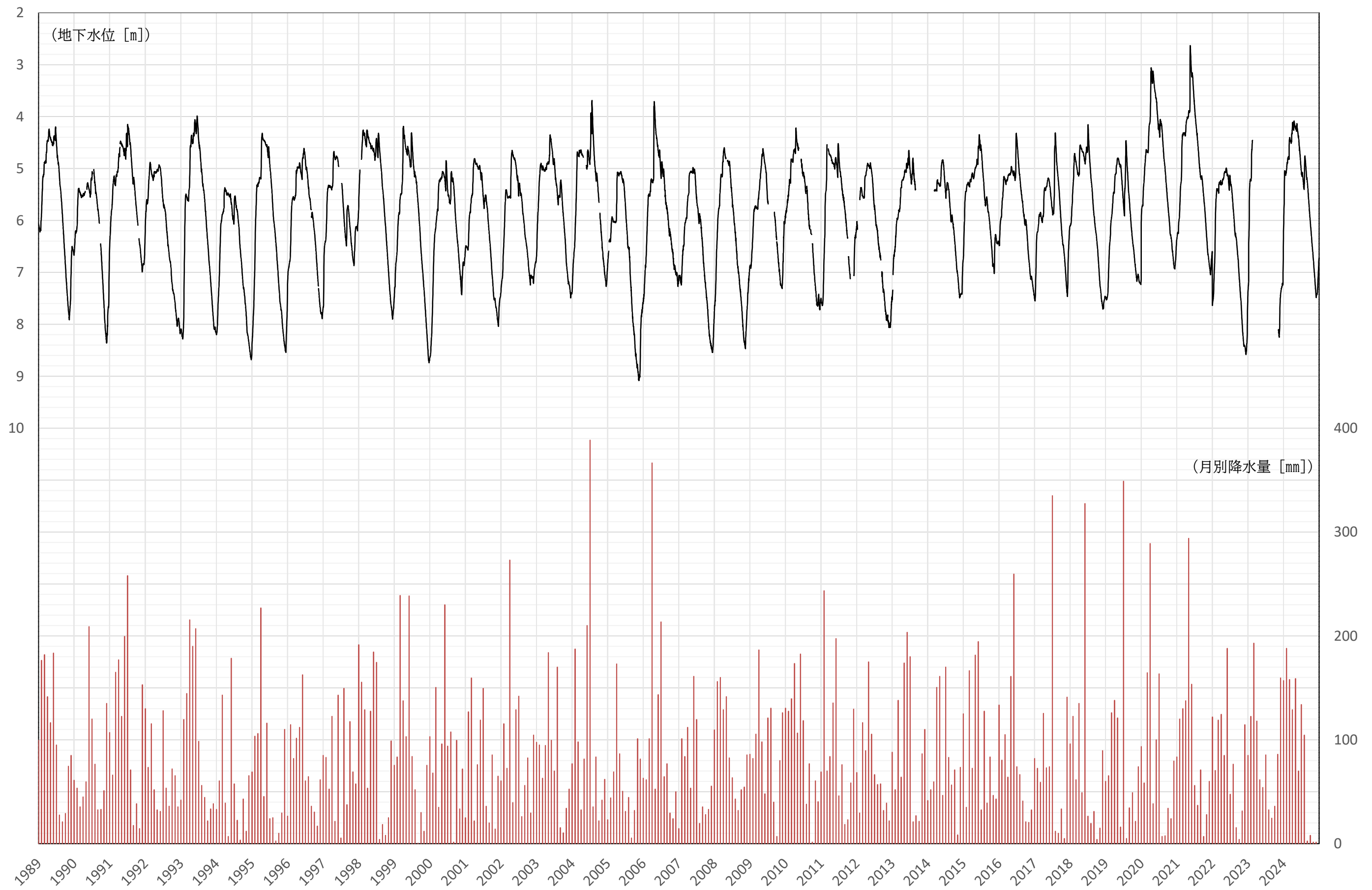
経年地下水位観測図 <島立観測井>
