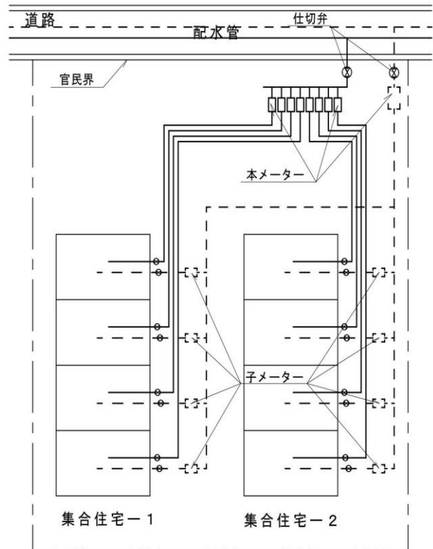
図ー２ 土地開発の方法、利用形態における水道施設の扱い
