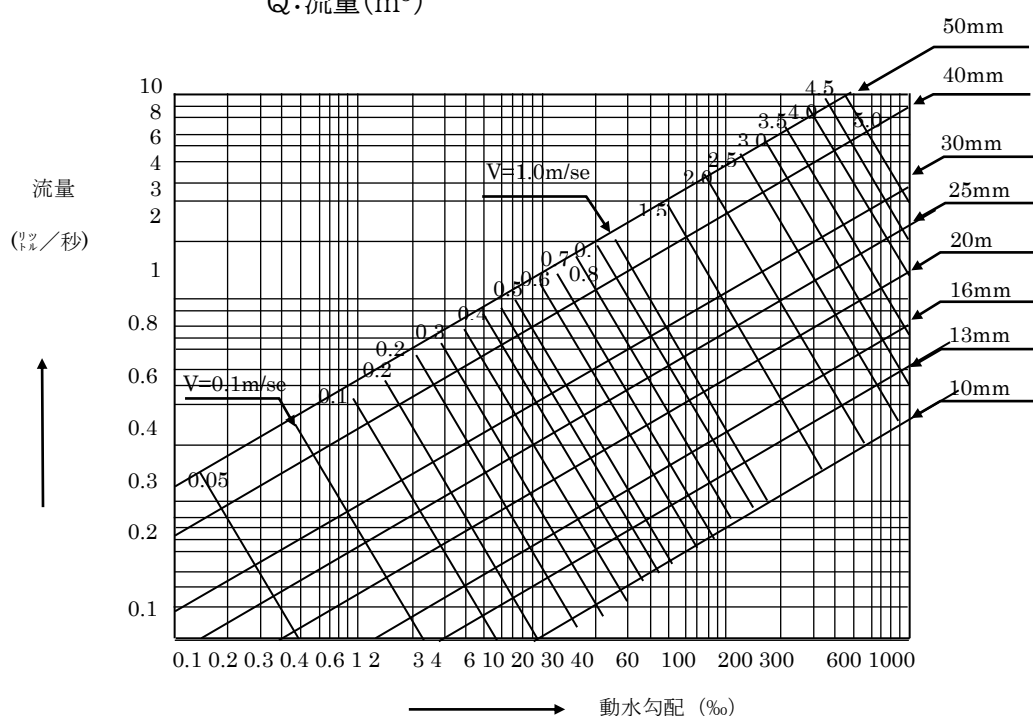
図-7 ウエストン公式による給水管の流量図
