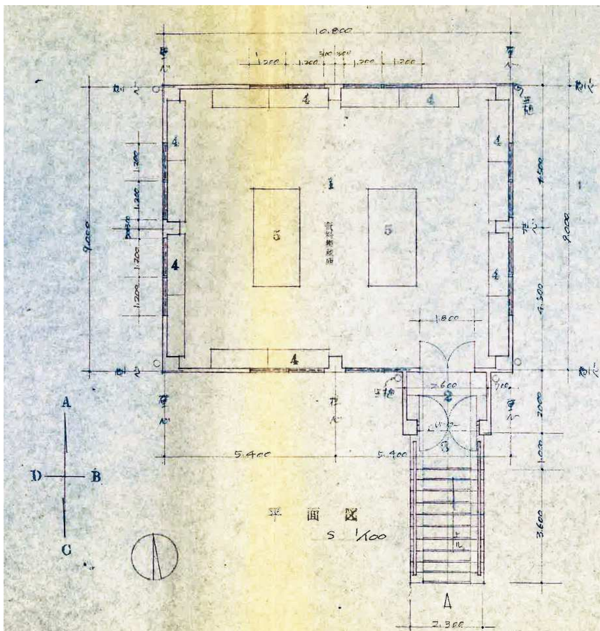
平面図
