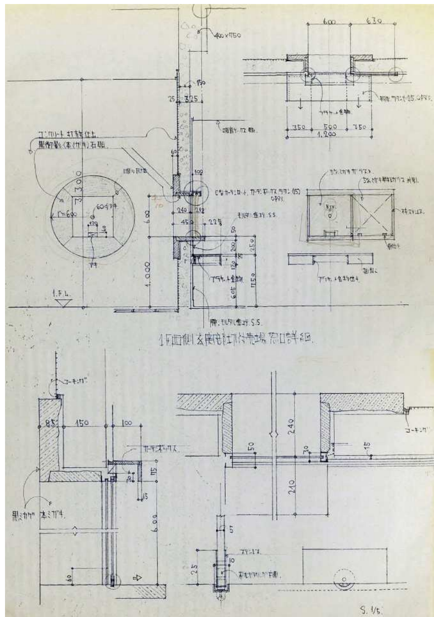
メインエントランス 切符売り場窓口詳細図
