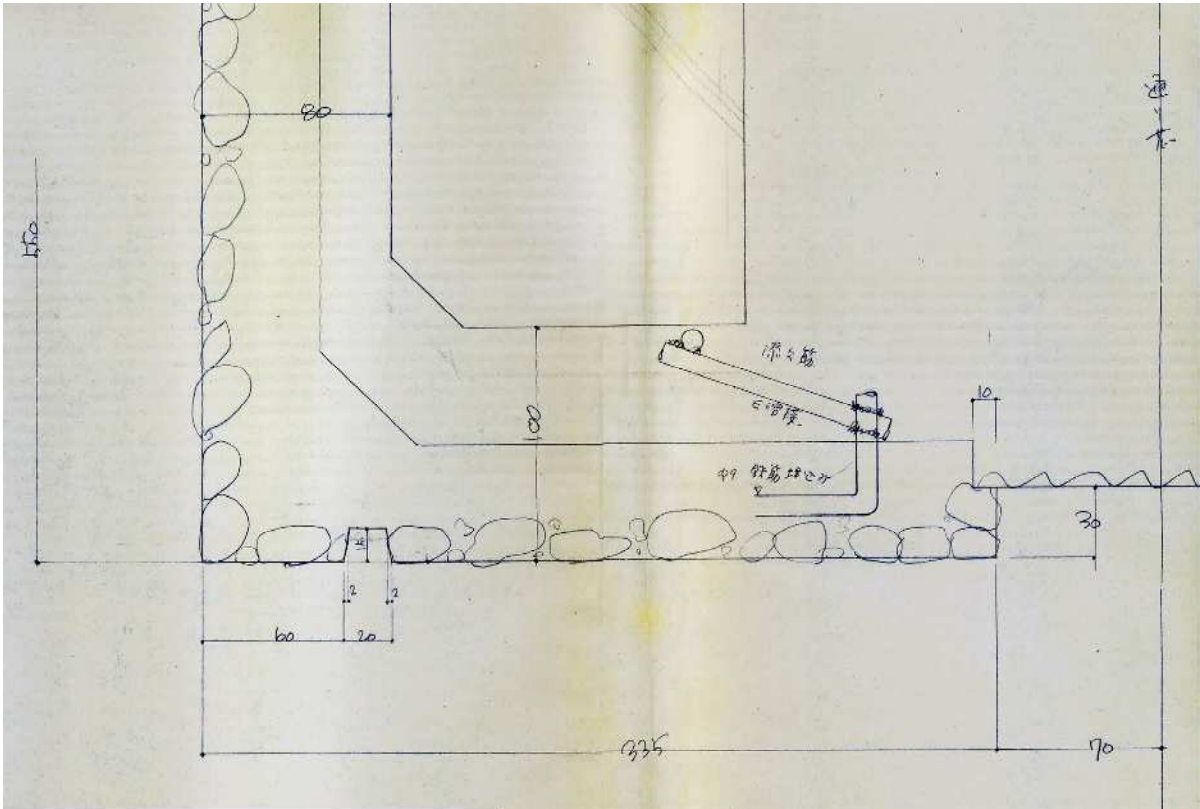
外壁プレキャストコンクリートパネル壁下端
