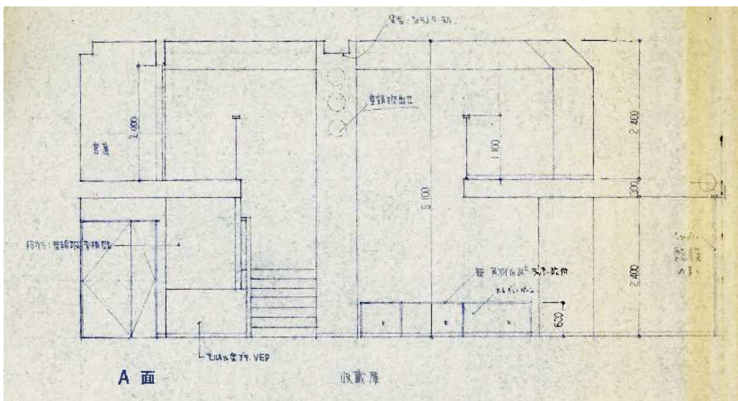
断面図 梁部分の天井を斜めにした事で、壁ガラリで天井裏換気が出来た。
