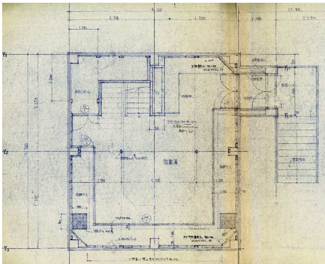
1 階平面図 貴重な古時計コレクションを収納するケースが造付けられた。
