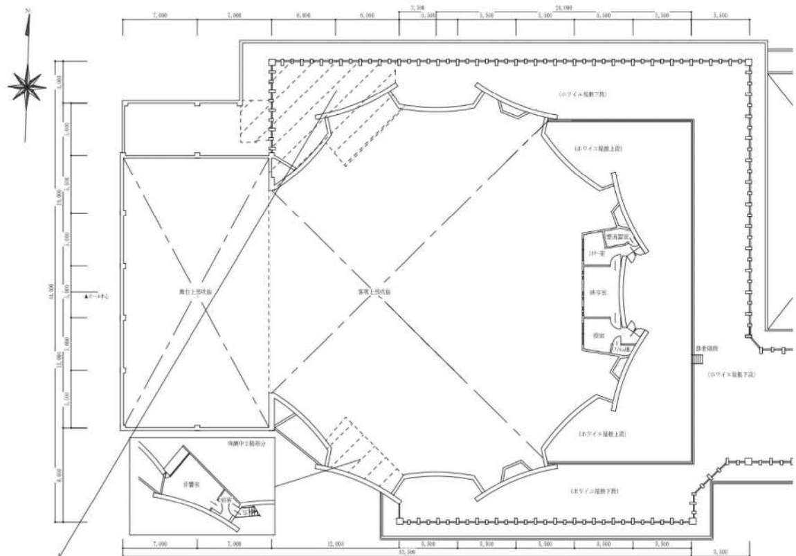
ホール棟2階平面図
