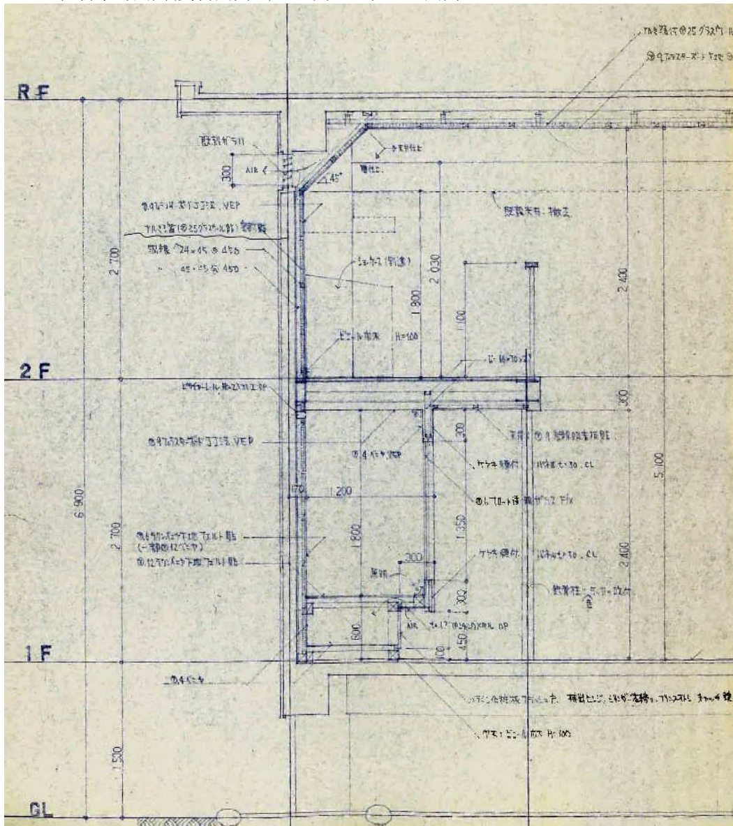
矩形図 天井を最大限上げて中二階を造り、壁・天井に断熱材を入れた。
