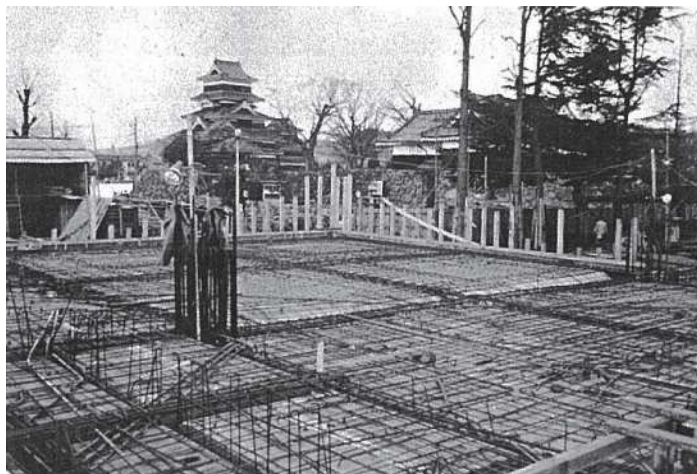
1 階スラブ配筋状況 (昭和41年(1966)3月28日撮影)
