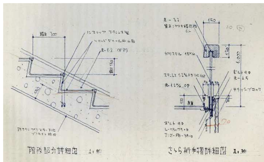
メイン階段詳細図
