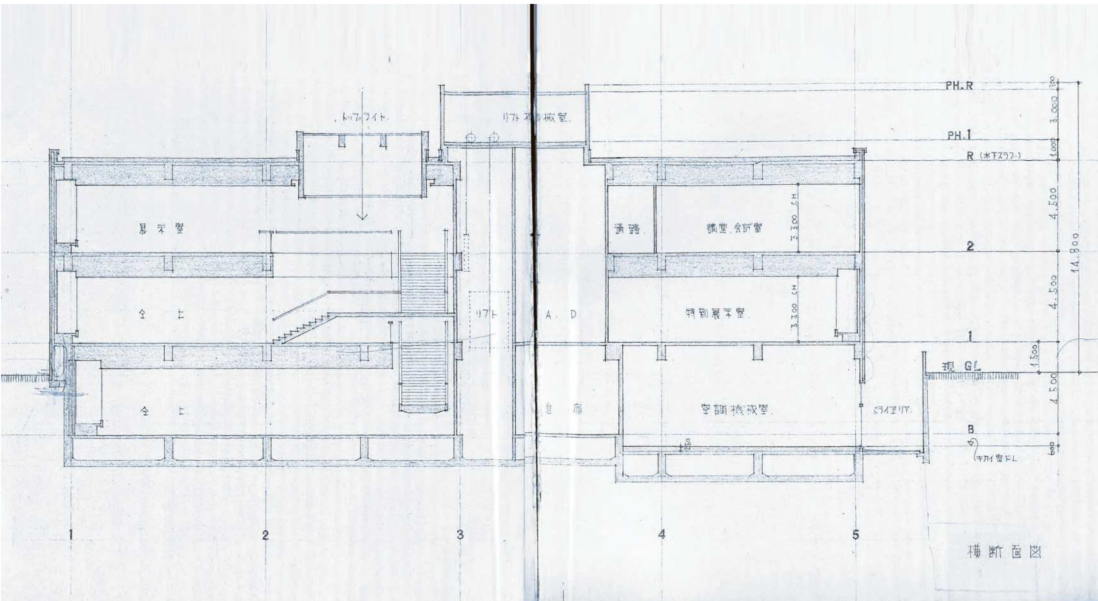
日本民俗資料館新築工事 横断面図
