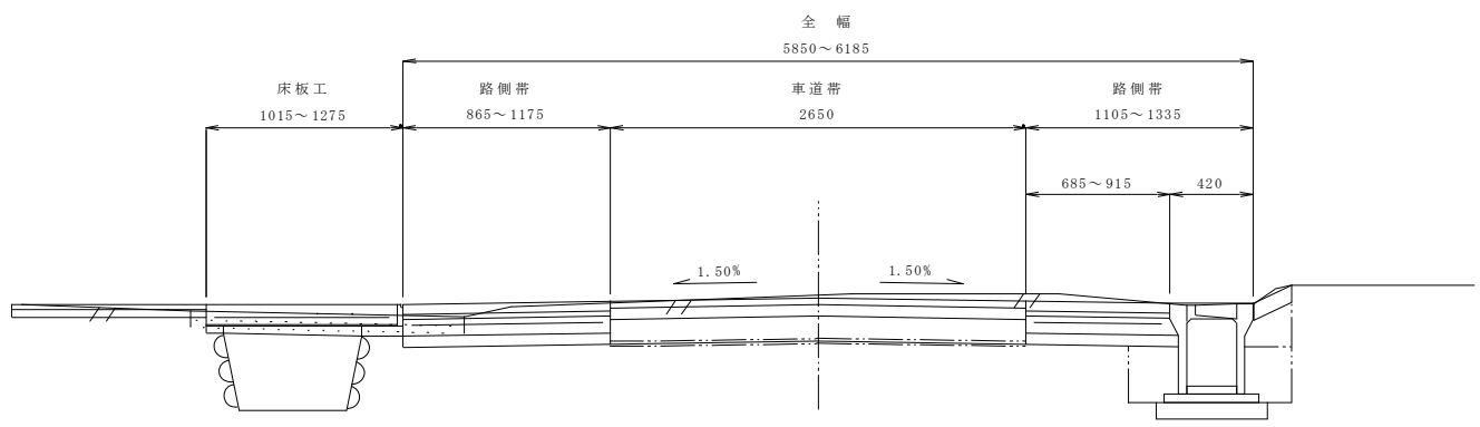
標準断面図
